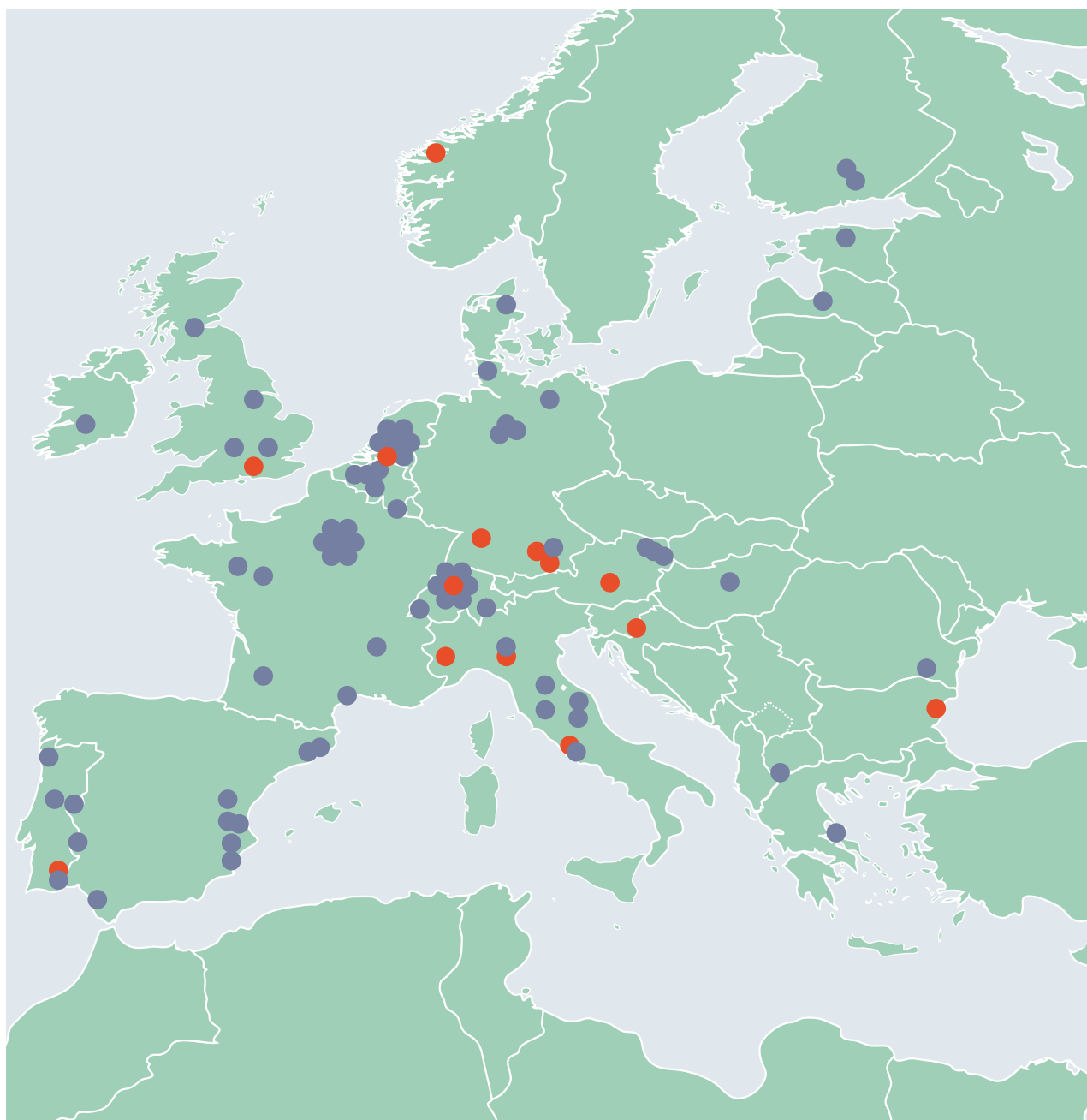
Mapa delle iniziative di miglioramento genetico biologico di piante (●) e animali (●) in Europa.
